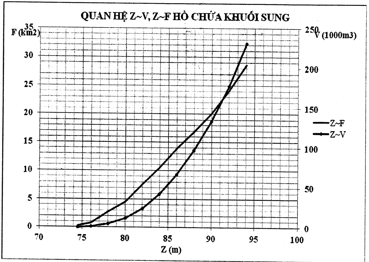
Hình 1: Đường đặc tính hồ chứa nước Khuổi Sung
