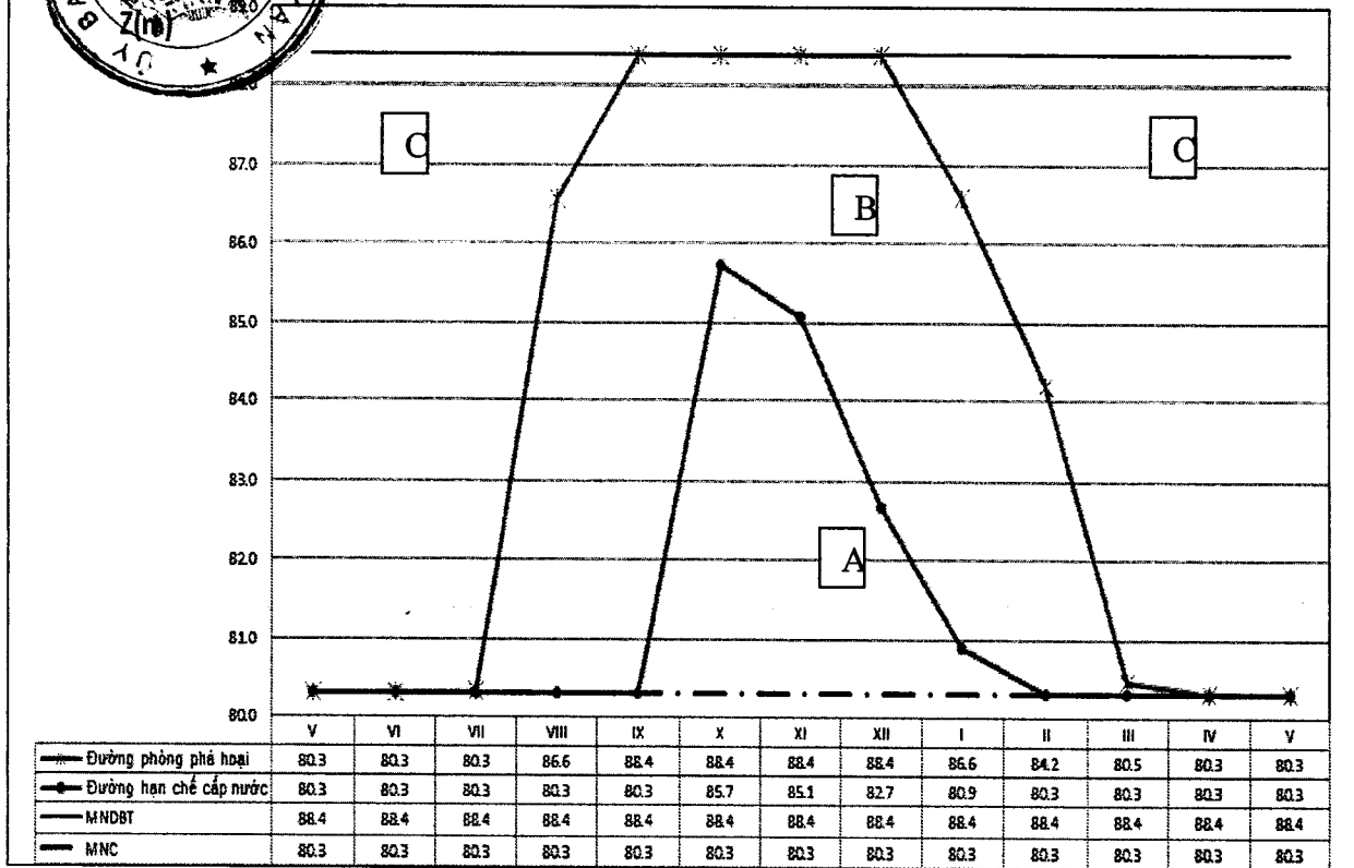
Hình 2: Biểu đồ điều phối hồ chứa nước Khuổi Sung
