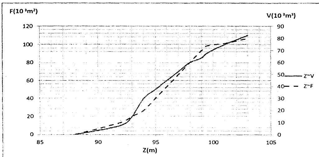
Hình 1: Đường đặc tính hồ chứa nước Tân Minh
